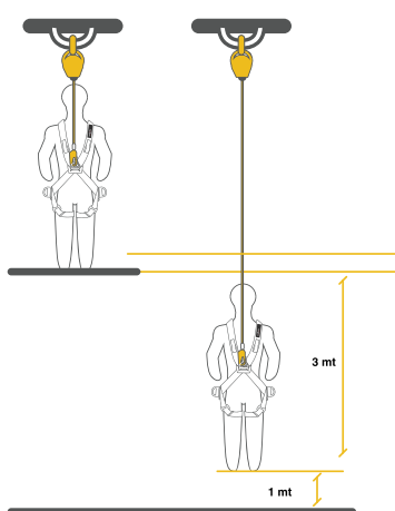
EFEECTO PENDULO
